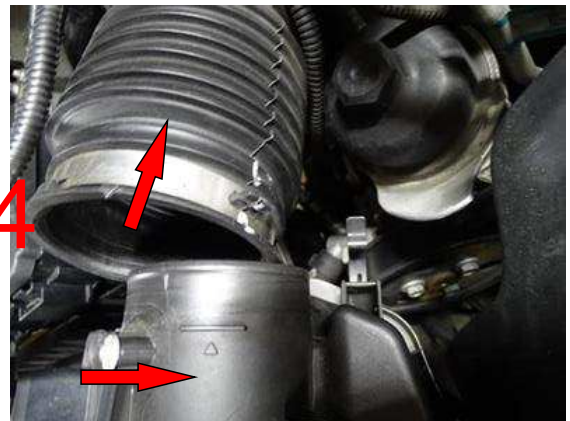
Schlauch und Deckel entfernen
