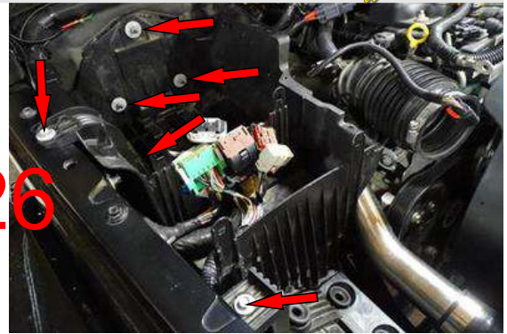
Schrauben lösen
