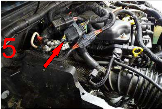
Kabelbaum zur Seite legen
