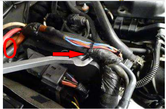
10 Klammern lösen
