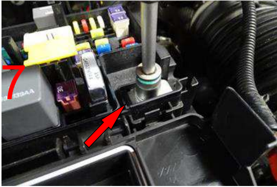
Stromzufuhr lösen
