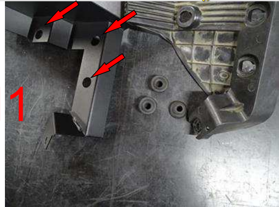
Gummis für Luftfilterkasten aus dem Originalteil in das Neuteil einsetzen
