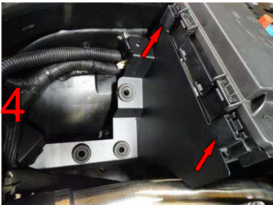
Halter von unten in den Sicherungskasten einklipsen
