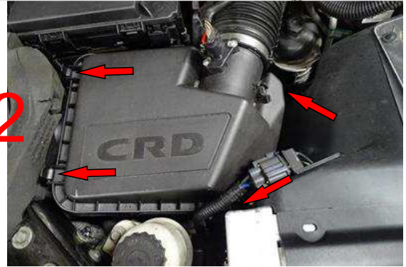
4 Klammern lösen
